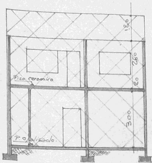
CORTE A-A
